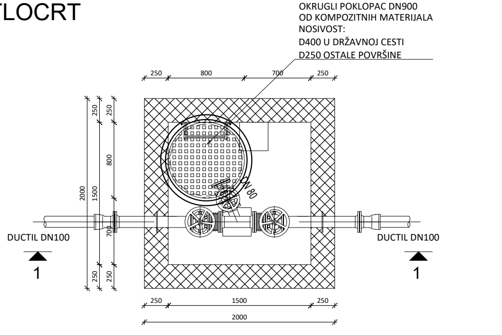
TLOCRT
