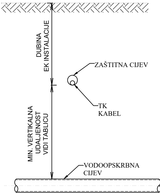
PRESJEK A - A
