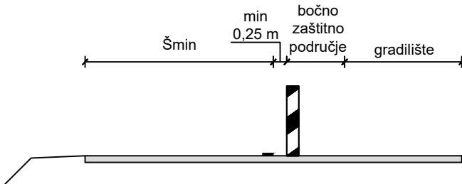
PRESJEK A - A
