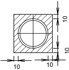
ZAŠTITNI BETONSKI BLOK L=2m
