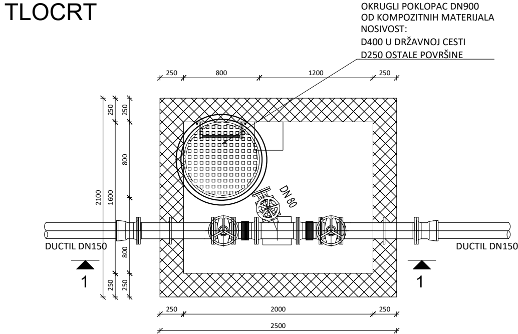
TLOCRT
